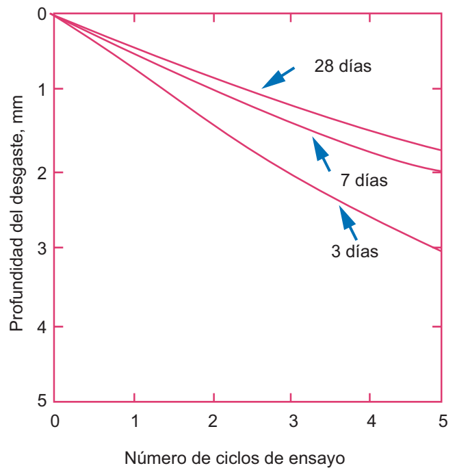
Figura No.6: Efecto del curado del concreto sobre la resistencia a la abrasión.
